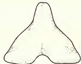
Coracias garrulus
